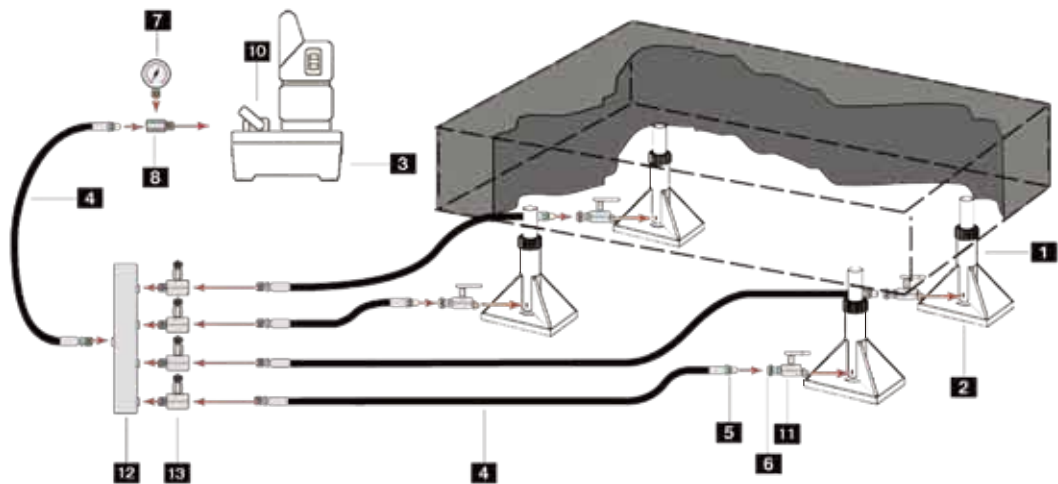
使用单作用液压油缸和方向控制阀的四点顶升配置
